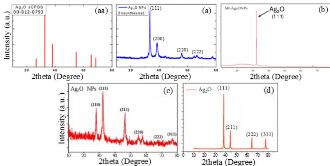
Hình 2 (a,b,c,d). Giản đồ nhiễu xạ XRD của các hạt nano \text{Ag}_2\text{O} ( \text{Ag}_2\text{O} NPs) theo các tài liệu [16-19].
