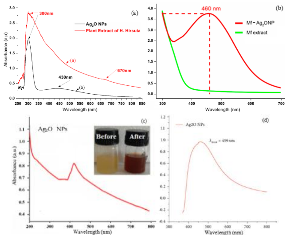
Hình 1 (a,b,c,d). Phổ hấp thụ UV-vis của các mẫu hạt nano \text{Ag}_2\text{O} ( \text{Ag}_2\text{O} NPs) theo các tài liệu [1-4].
