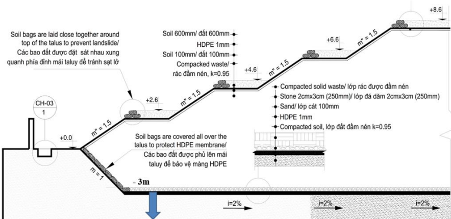
Hình 4. Mặt cắt điển hình của thiết kế bãi chôn lấp
