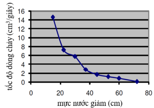
Hình 7. Mối quan hệ giữa tốc độ dòng chảy và mức nước giảm.
