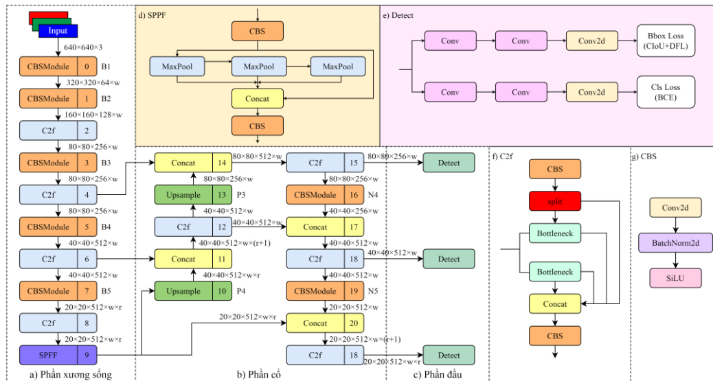
Hình 2. Cấu trúc của mô hình YOLOv8 [18].
